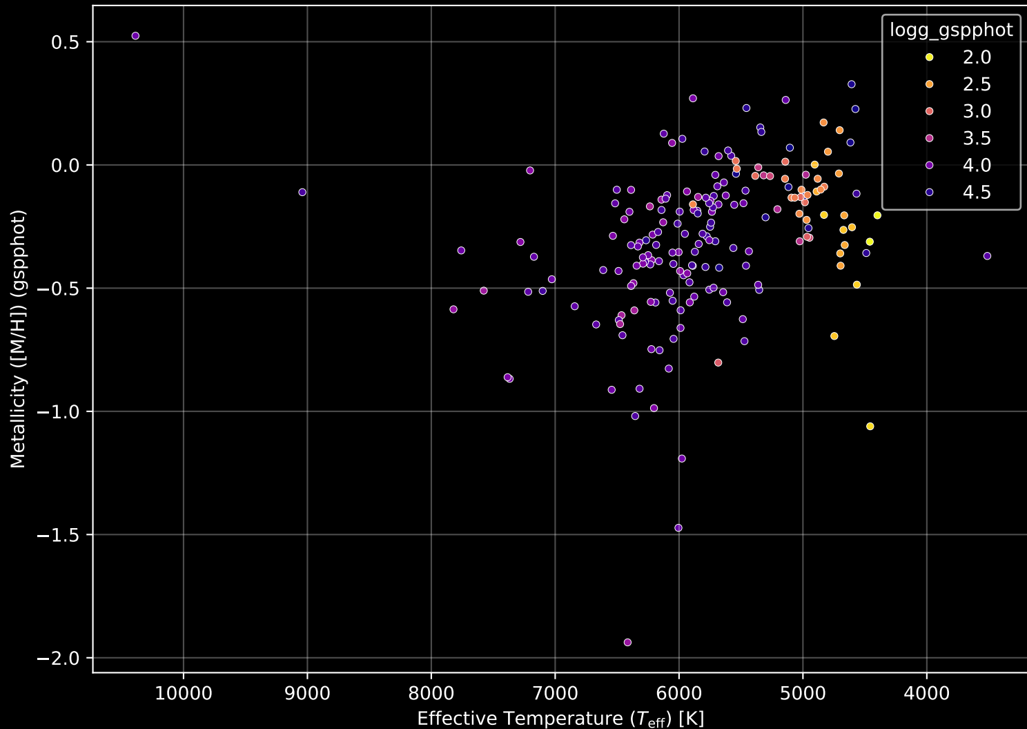
GALAH DR4 Field: [7222] Stellar Population Parameters (n= 191)
