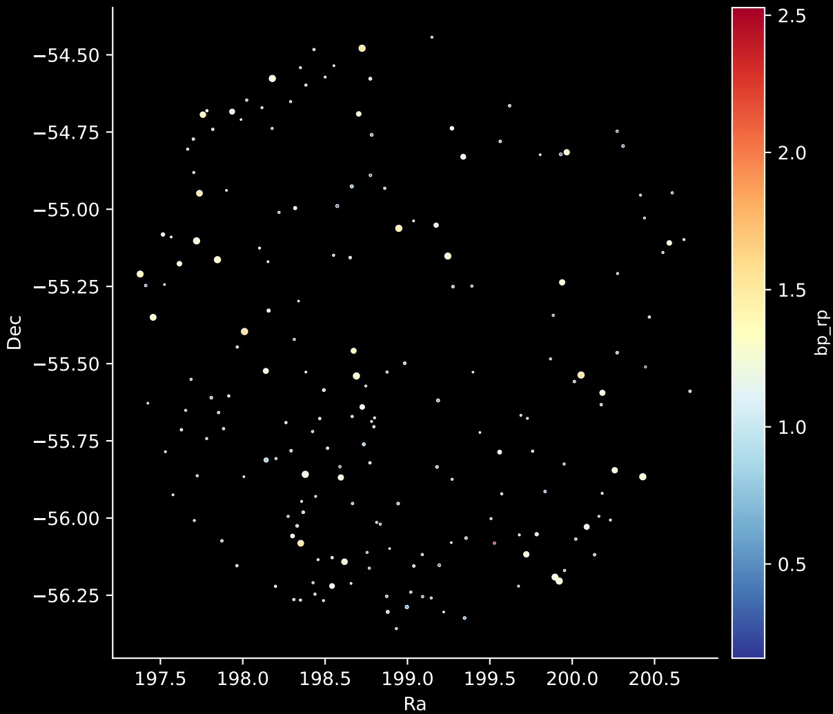
GALAH DR4 Field: [7222] Stars: 191
